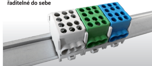
Smyčkování rozváděčových skříní
