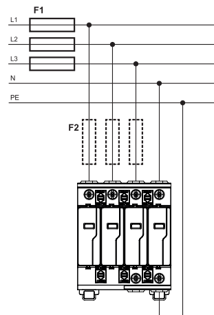
TN-S
