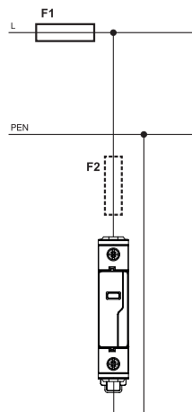
TN-C
